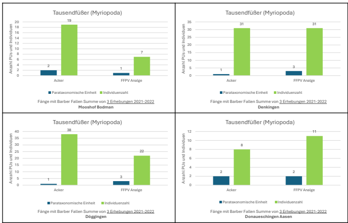
Abbildung 44: Kumulierte Fänge von Tausendfüßern in drei Fangperioden 2021–22 an den vier Standorten (Säule blau max. Anzahl der PU Artengruppen, rechte Säulen Anzahl Individuen).
