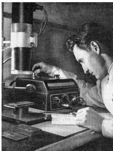
Abb. IV.2: Bestimmung der Dicke von Lackschichten durch Rückstreuungen mit ^{204}\text{Th} allium
