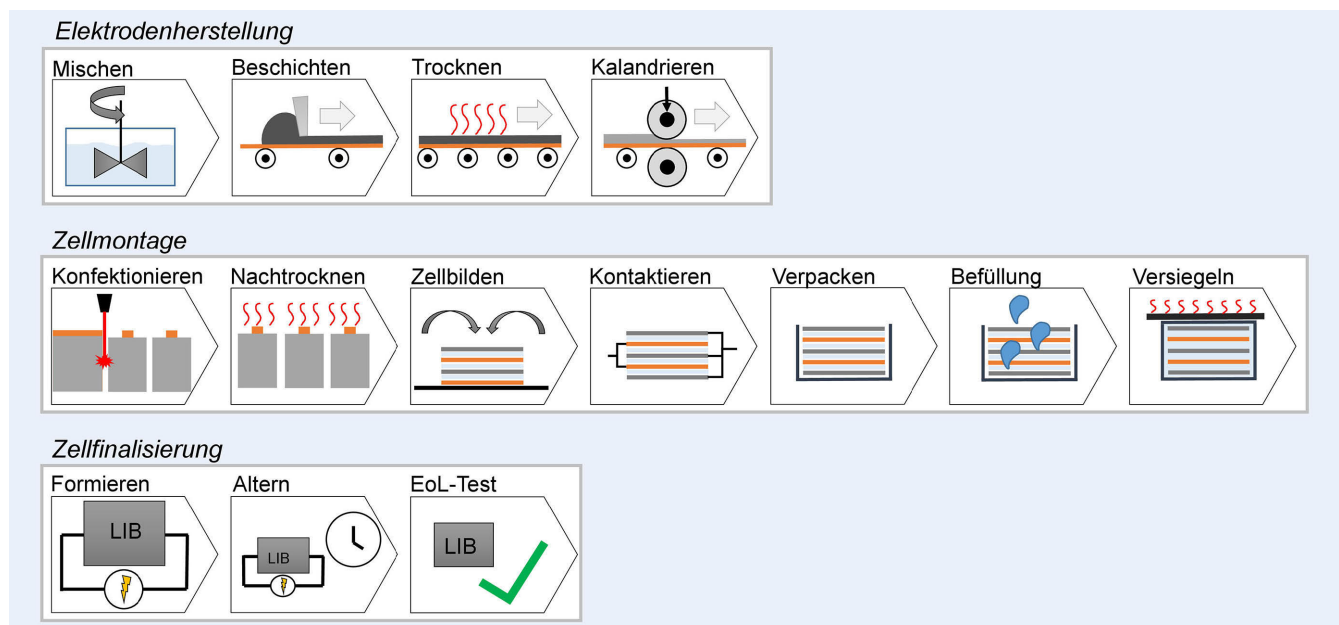
Bild 1. Prozesskette der Batteriezellproduktion von Lithium-Ionen-Batteriezellen. Grafik: Simon Otte
