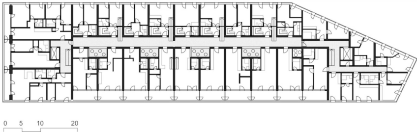
Abb. 4: Der Grundriss des Integrativen Bauprojekts am ehemaligen Blumengroßmarkt (IBeB) zeigt verschieden große und unterschiedlich geschnittene Wohnungen. Die über Lichthöfe beleuchtete rue intérieure (in grau) ist als gemeinschaftlicher Begegnungsraum konzipiert, eigene zeichnerische Darstellung.
