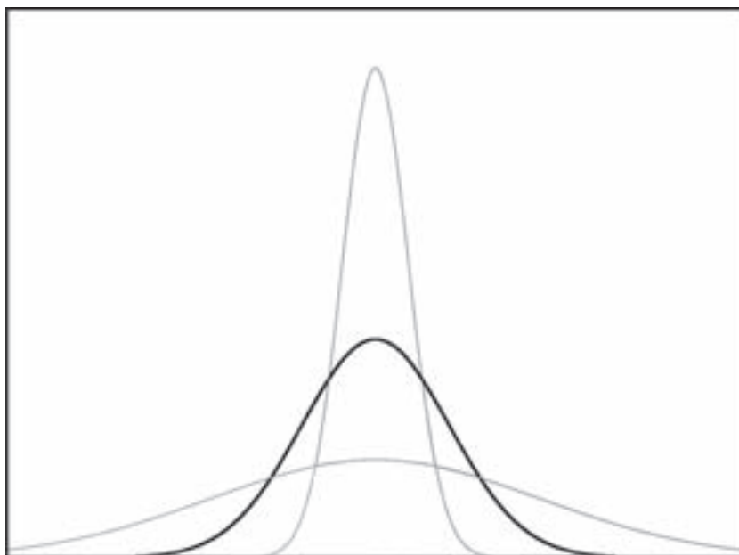
Abb. 1 – Gauß'sche Verteilungen
