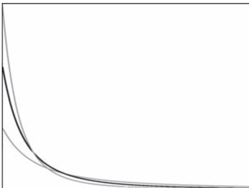
Abb. 2 – Schiefseitige Verteilungen
