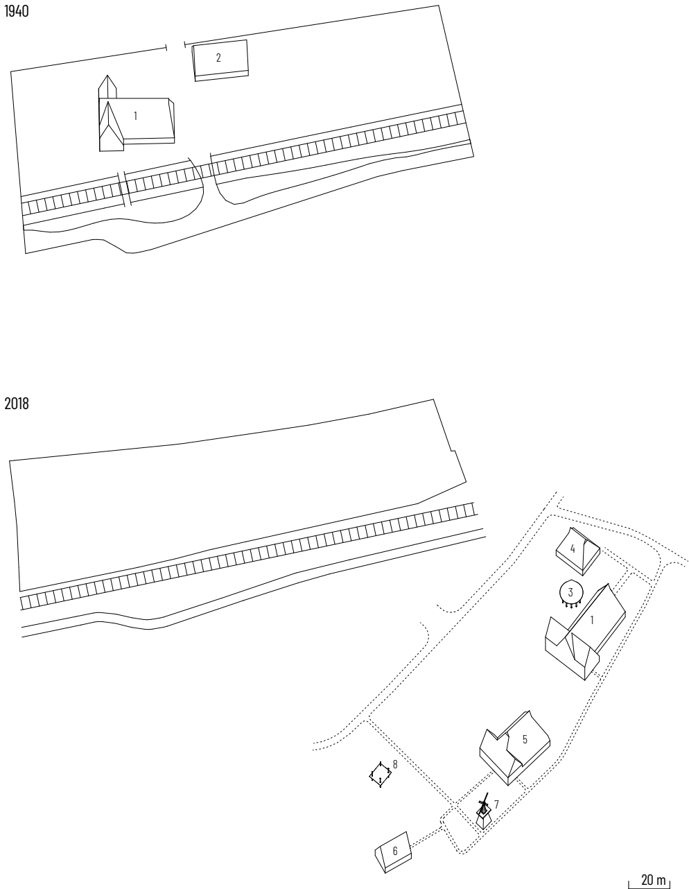
4-24 Genordete Grundriss-Axonometrie 1940 (oben) und 2018 (unten links vor Ort; unten rechts im Museum). M 1:2.500. Lüder, Herrera, 2018. Datengrundlage: Wolf 1979; © Geobasis-DE/LVermGeo SH 2015 ALKIS; Aufmaß.
