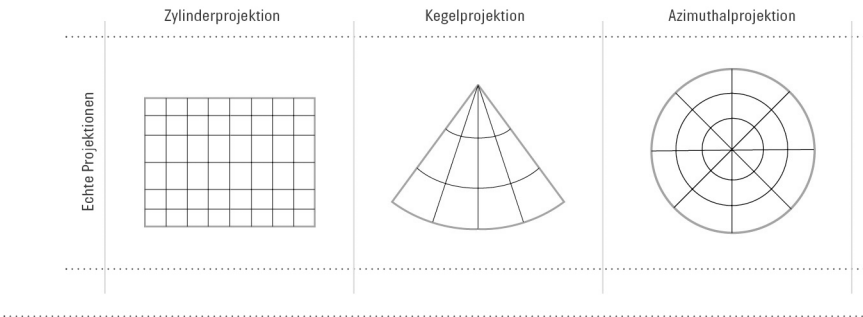
Abb. 23: JMS. Beispiele von Projektionsarten und deren Umrissformen. Nach: Canters und Declair (1989, S. 29)
