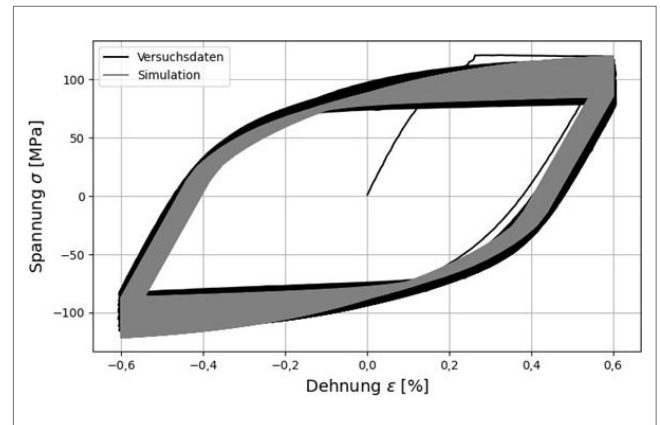
Bild 14 Vergleich der Hysteresen aus dem Versuch V02_e06_längs bei \varepsilon_{a,T} = 0,6 \% mit den Hysteresen des schadigungsabhängig modifizierten Werkstoffmodells. Grafik: Fraunhofer LBF
