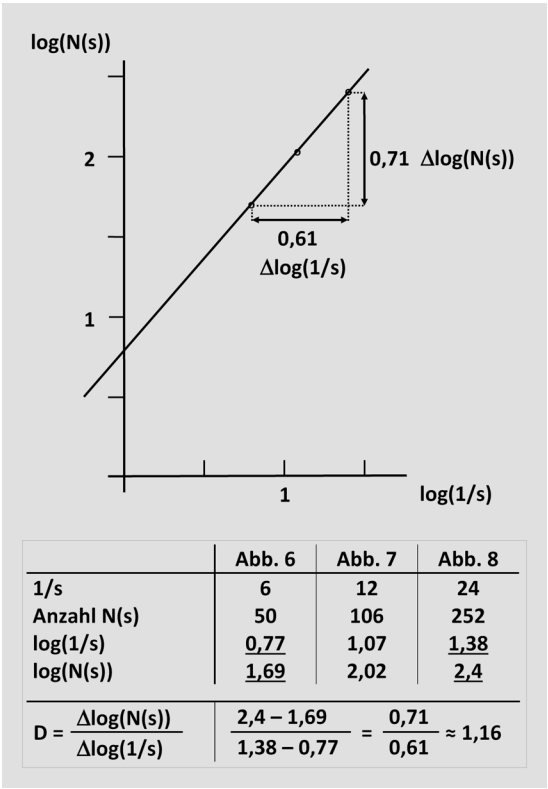
Abb. 9: Bestimmung der Box-Dimension
