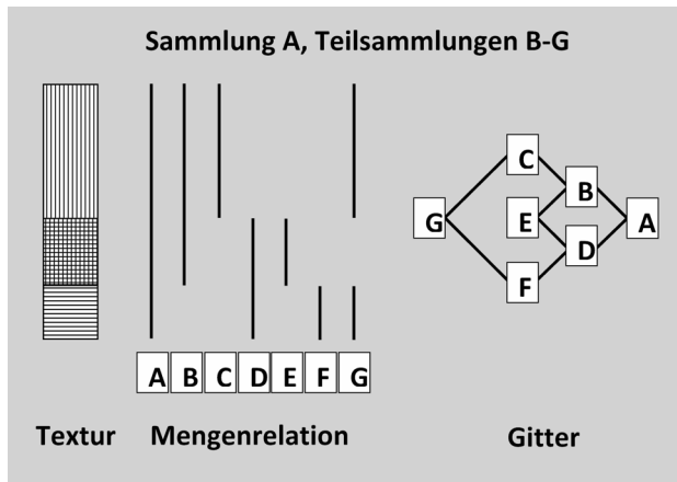
Abb. 3: Dekomposition einer Sammlung mit polyzentrischer Struktur
