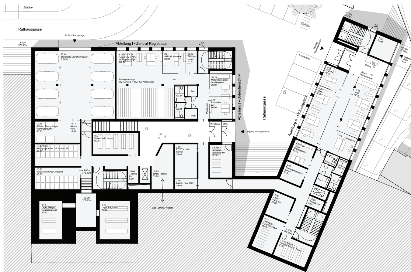
Grundriss Sockelgeschoss
