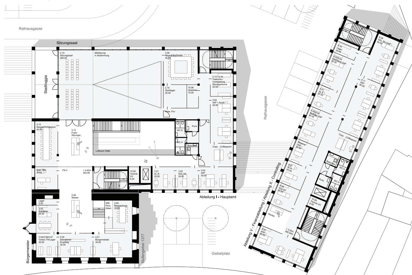
Grundriss 1. Obergeschoss
