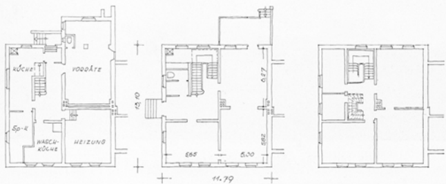
Abb. 148. Keller-, Erd- und Obergehoßgrundriß des Kopfbauers der gleichen Hausreihe
