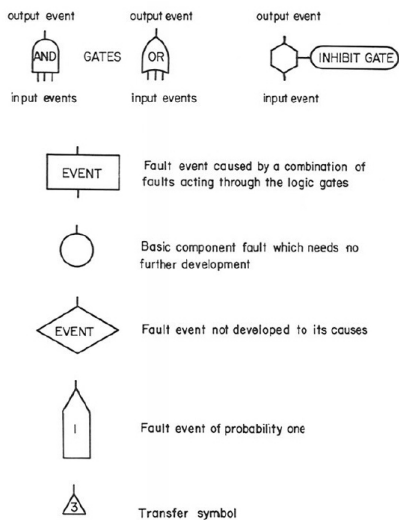
Abb. 6 Schaltoperatoren und Schaltdiagramm einer Fehlerbaumanalyse
