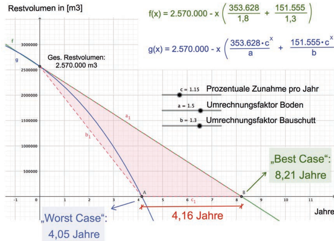
Abbildung 41 Mathematische Langzeitsimulation zur Bewertung der Entsorgungssicherheit [Eigene Berechnung mit GeoGebra (CAS-System), 29.12.2021]
