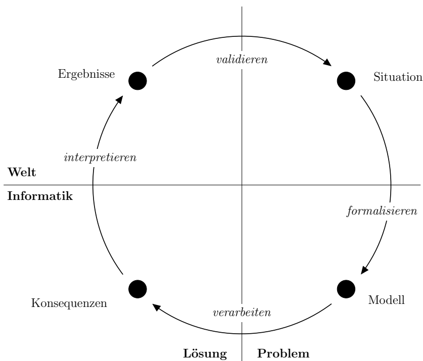
Abbildung 2.1: Informatischer Modellierungskreislauf 12
