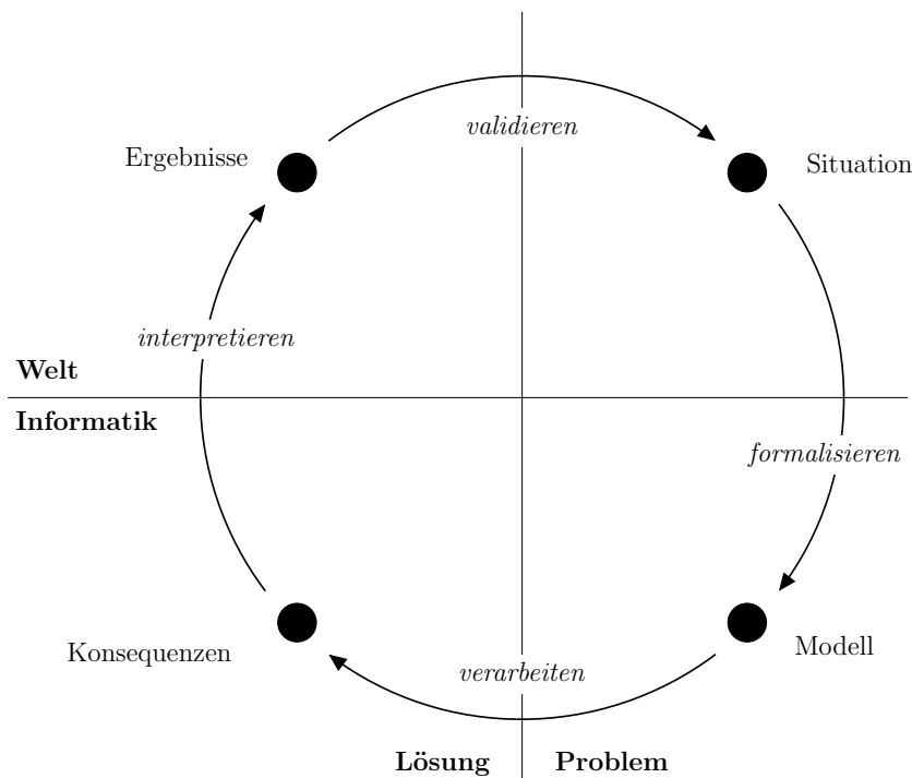
Abbildung 2.1: Informatischer Modellierungskreislauf 12
