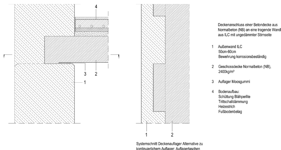
Abb. 54: Deckenanschluss einer Betondecke aus Normalbeton (NB) an eine tragende Wand aus Infralichtbeton (ILC) mit ungedämmter Stirnseite © ILC 494
