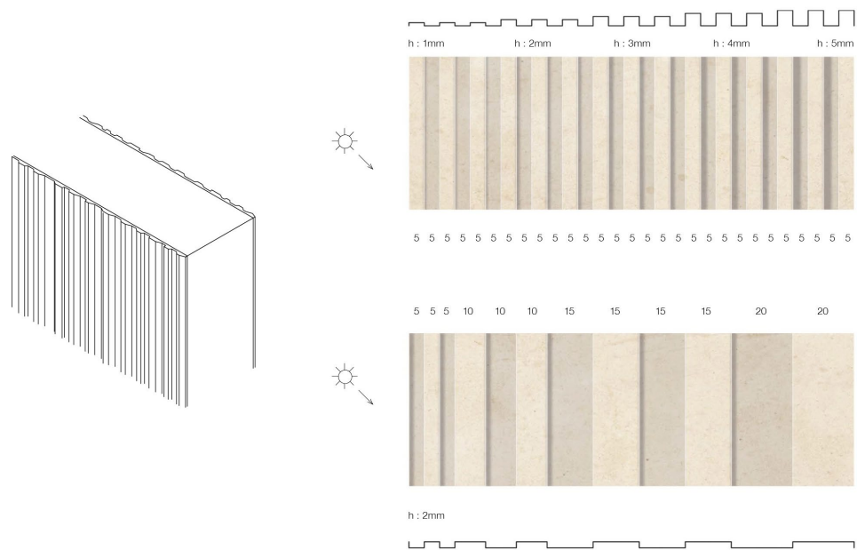
Abb. 85: Individualisierte Oberflächengestaltung des mehrschichtigen Wandaufbaus © TU Dortmund, Lehrstuhl Baukonstruktion, Juniorprofessur REB (Lowin)
