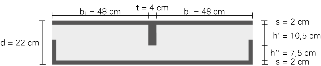
Abb. 65: optimierter Wandquerschnitt © ILEK 529
