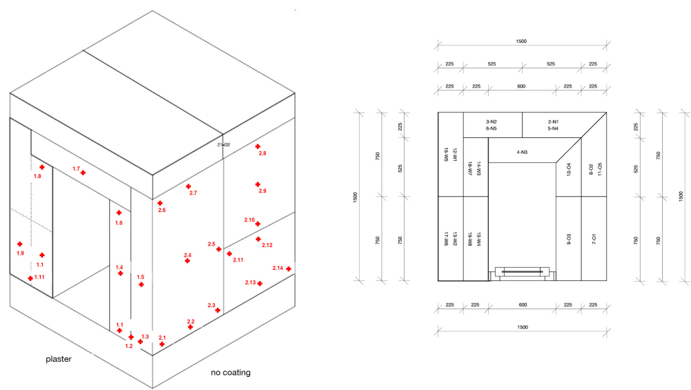
Abb. 83 Konzipierung des Demonstrators © TU Dortmund, Lehrstuhl Baukonstruktion, Juniorprofessur REB (Lowin)
