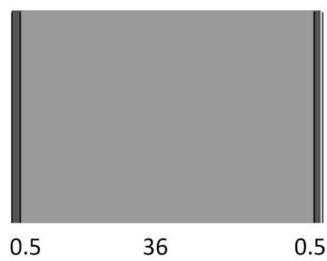
Abb. 74: Schematische Darstellung des hybriden Bauteils mit einem Querschnitt von 37 cm. Eigene Darstellung
