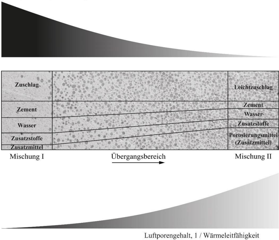
Abb. 61: Eigenschaftsänderungen der Betongemische durch Dichteanpassung 517 © ILEK
