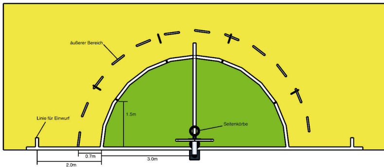
Abbildung 2: Maße für den Seitenbereich des »Baskin«-Spielfelds
