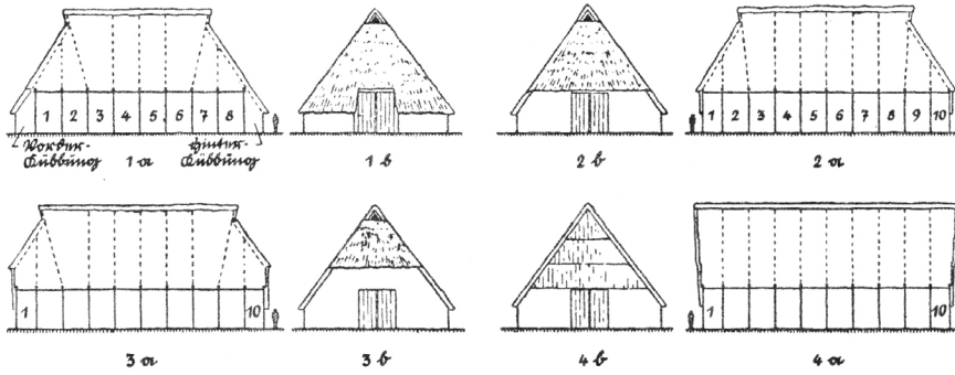
Fig. 26 1 Kollmoosalm über 8 baul, beide vordere und hintere Pfostenkriibbing. 2 Kollmoosalm über 10 baul, keine Pfostenkriibbing. 3 Krippenmoosalm. 4 Kollmoosalm
