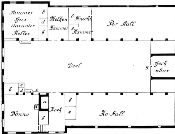
Grundriß
