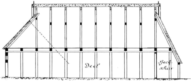
Längenschnitt
