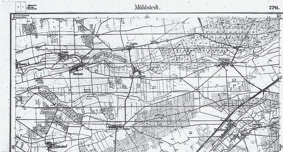
Projektierte Flugstreifen in Flughöhe von 1000m. f: 20cm, für den Aufnahme-Maßstab 1:5000 Seitliche Überdeckung 30%
