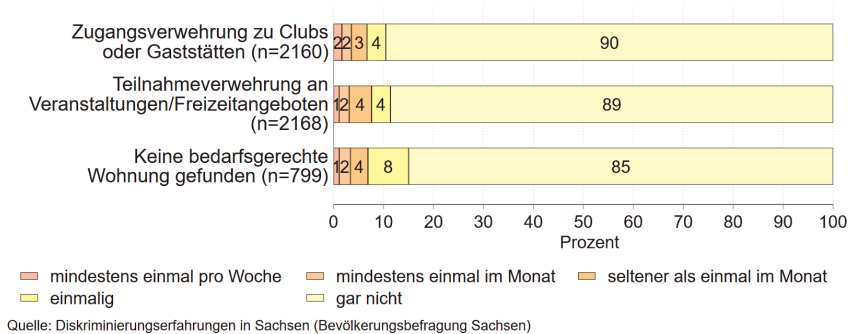
Abbildung 32 Materielle Benachteiligung
