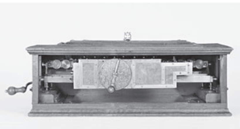
Abb. 3: Vier-Spezies-Rechenmaschine von Gottfried Wilhelm Leibniz, Ende 17. Jahrhundert
