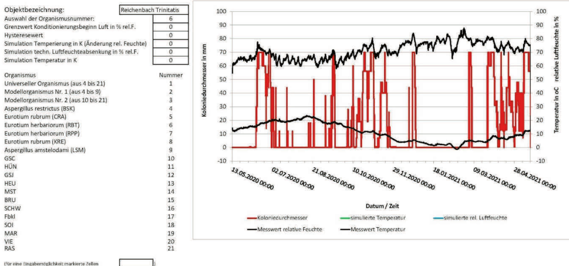
Abb. 18 Reichenbach Trinitatiskirche, Korrelation der Raumklimaaufzeichnungen [schwarz] aus der Orgel der Kirche mit den mikrobiologischen Wachstumsbedingungen [rot]. (Ohne Belang für die Simulation ist der Umstand, dass die Heizung während der Beobachtungszeit ausgefallen war).
