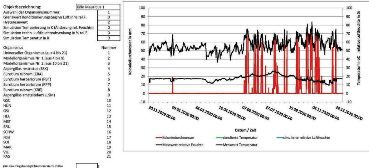
Abb. 27 Klimadiagramm für St. Mauritius in Köln mit den simulierten Wachstumsbedingungen. Mit dem signifikanten Ansteigen der relativen Luftfeuchte im Juni 2020 auf Werte über 60% rel. F. verbesserten sich die Wachstumsbedingungen sprunghaft, da auch die Temperatur anstieg und zumeist Werte über 15°C herrschten. Von November 2019 bis Mitte März 2020 lag die Raumtemperatur in Folge einer kontinuierlichen Beheizung konstant bei 18°C, während sie im November und Dezember 2020 schwankte und zweitweise auf 10°C sank.
