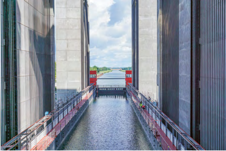
Abb. 6: Schiffshebewerk Lüneburg, Blick auf den Trog im westlichen Förderportal, Foto 2019.
