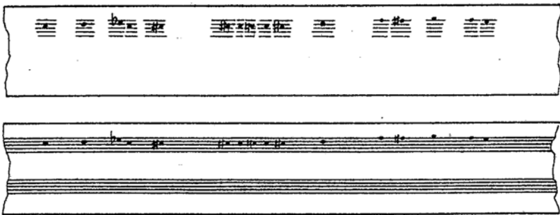
Abbildung 2.11: Das Rhythmusband.
