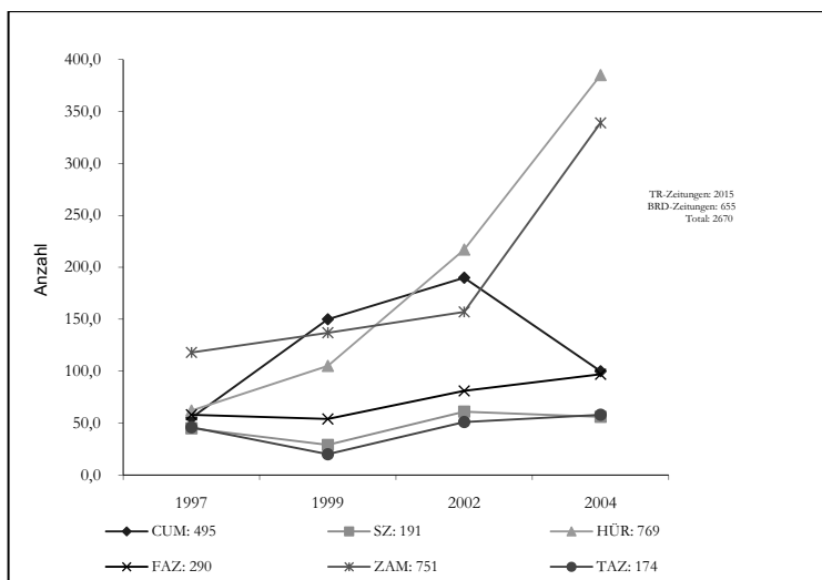
Abb. 1. Artikelanzahl & Jahr
