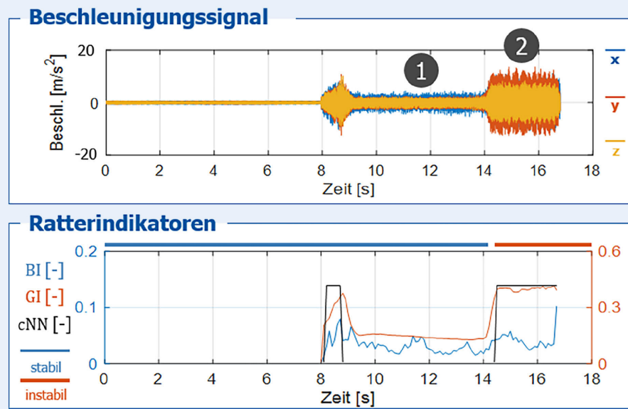
Bild 3. Rattererkennung bei hochfrequenten Schwingungen. Grafik: WZL
