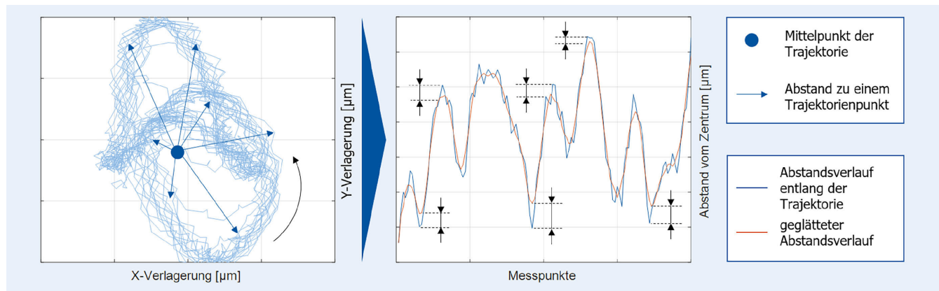
Bild 5. Vorgehen zur Bestimmung des Glattheitsindikators (GI). Grafik: WZL
