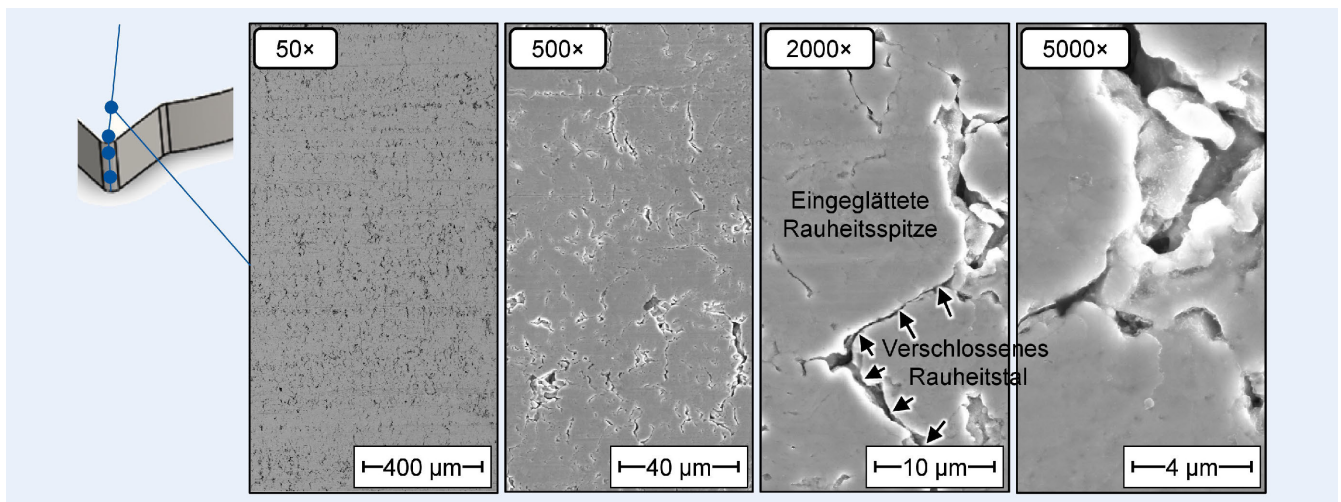
Bild 8. Ansicht der kaltgewalzten Bandoberfläche mittels Sekundärelektronenmodus. Grafik: MTI
