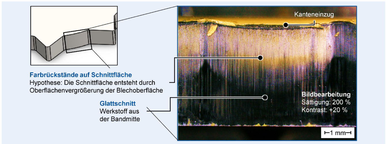
Bild 4. Nachweis der Oberflächenvergrößerung durch Analyse von Merkmalen, die ehemals auf der Bandoberfläche vorlagen. Grafik: MTI
