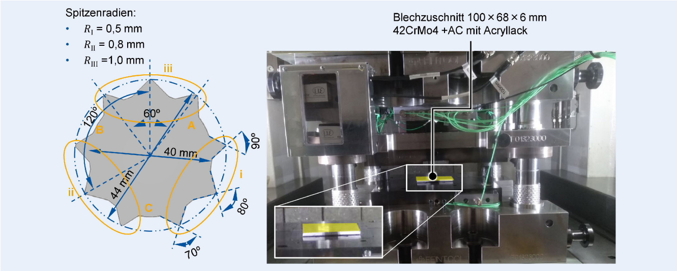
Bild 3. Verwendete Geometrie und Versuchsaufbau im Feinschneidwerkzeug. Grafik: MTI
