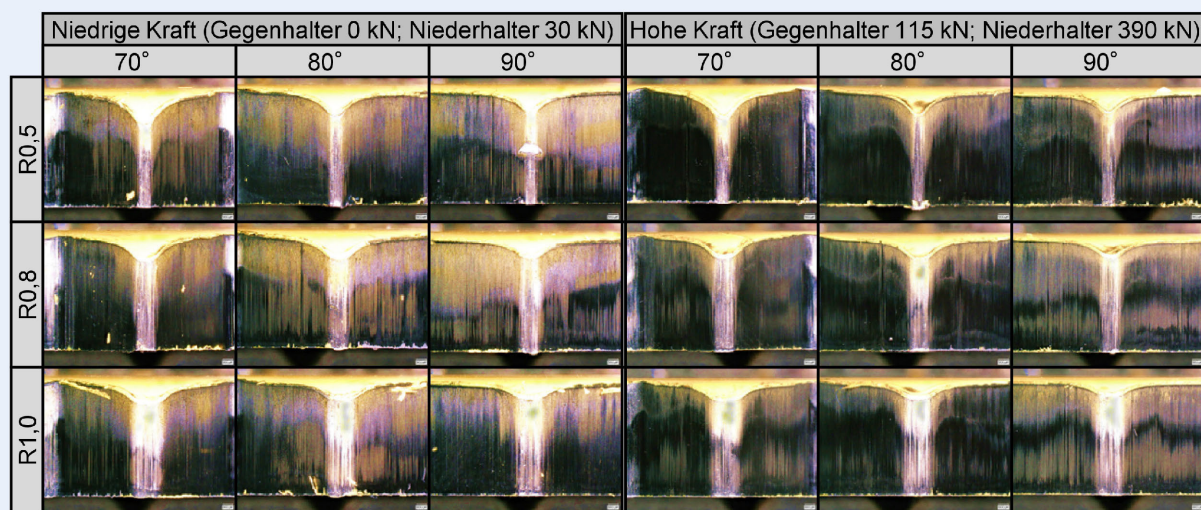
Bild 5. Gegenüberstellung der Auswirkung von Geometriefeatures (Spitzenradius R und Eckenwinkel) und Prozesskraft auf die Oberflächenvergrößerung der Bandoberfläche auf die Schnittfläche. Grafik: MTI
