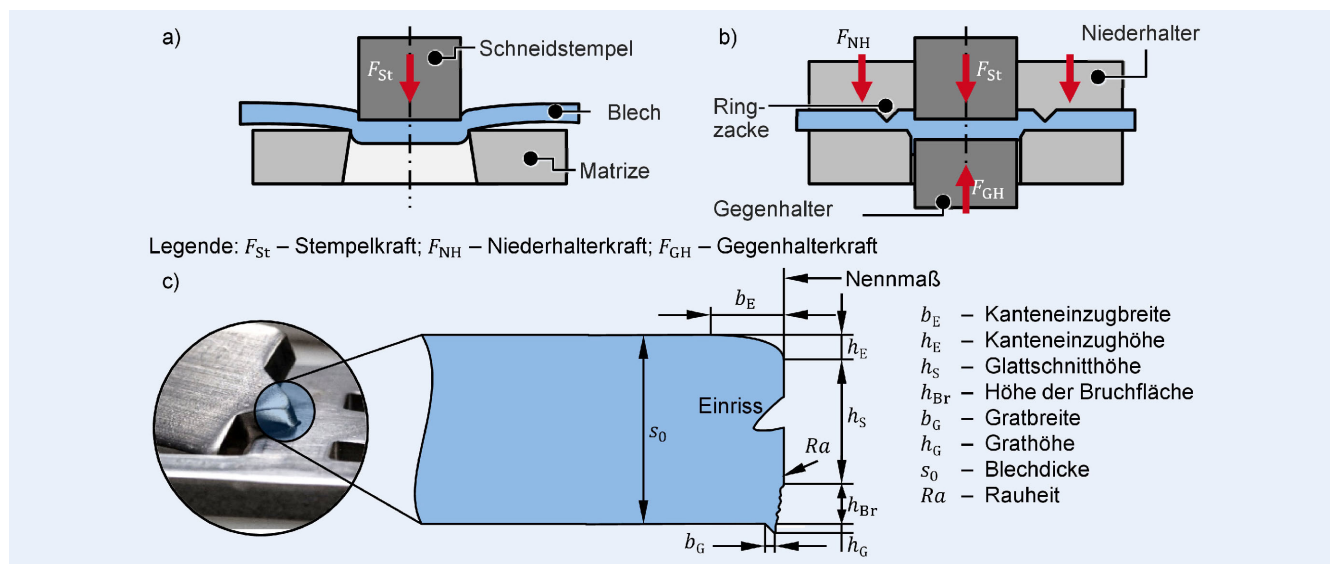
Bild 1. Prinzip a) des Normalschneidens im Vergleich zum b) Feinschneiden und c) Definition von Schnittflächenmerkmalen. Grafik: MTI nach [2]
