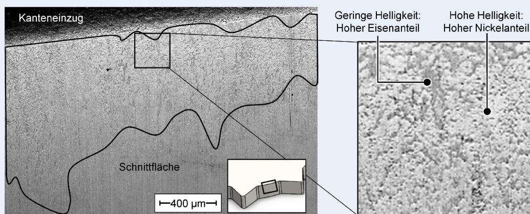
Bild 6. Nachweis von Nickel von der Bandoberfläche kommend auf der Schnittfläche mittels Rückstreuelektronen. Grafik: MTI
