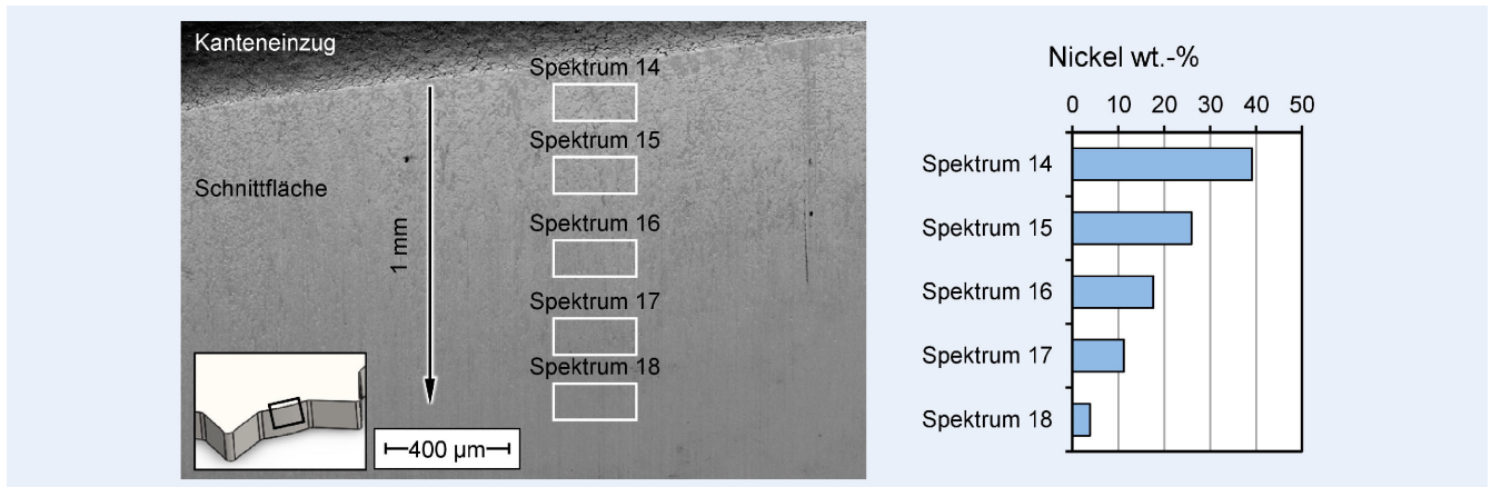
Bild 7. Nachweis von Nickel auf der Schnittfläche mittels EDX (energy dispersive X-ray spectroscopy)-Messung. Grafik: MTI
