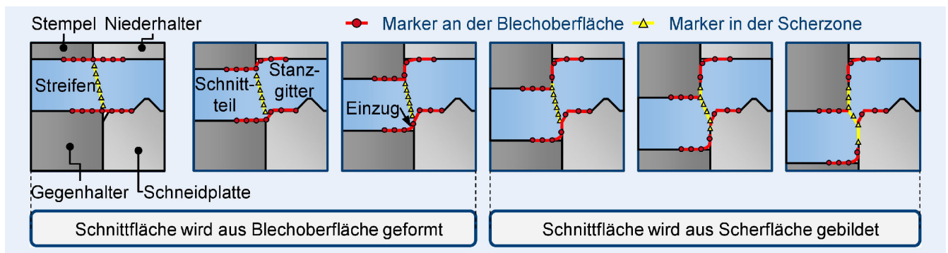
Bild 11. Modellvorstellung des Trennmechanismus beim Feinschneiden mit virtuellen Markern auf der Bandoberfläche (Kreis) und in der Scherzone (Dreieck). Grafik: MTI
