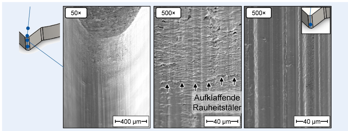
Bild 10. Ansicht der Glattschnittfläche unterhalb des Kanteneinzugsbereichs und auf der Gratseite mittels Sekundärelektronenmodus. Grafik: MTI
