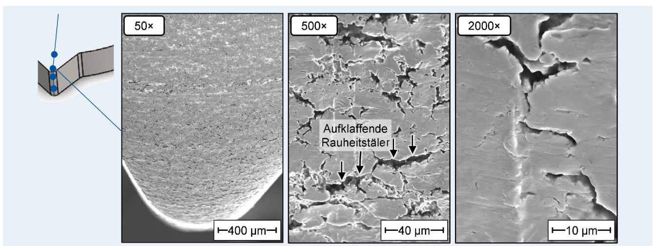
Bild 9. Bereich des Kanteneinzugs an einem Schnittteil auf der Oberseite mittels Sekundärelektronenmodus. Grafik: MTI
