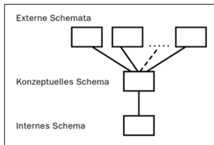
Abb. 10: ANSI/X3/SPARC-Datenbankarchitektur
