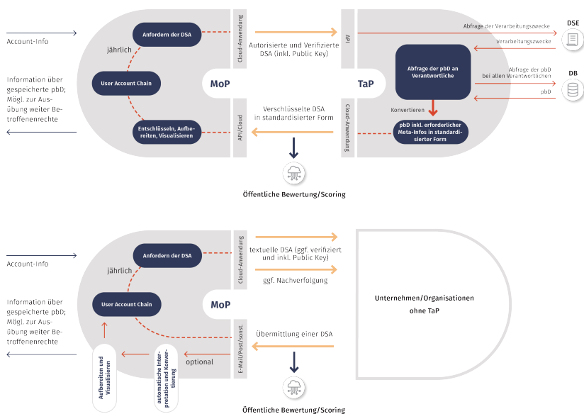
Abb. 2. Schematische Darstellung des PIMS bestehend aus der Bürger:innen-Einheit Monitoring Tool for Personal Data (MoP) und dem Komplementärssystem für DH: Tool for automated Data Self-Disclosure Request Processing (TaP).
