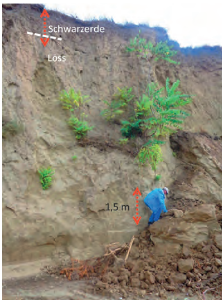
Abb.II.7.2 Lössprofil von Isaccea (nördliche Dobrudscha)
