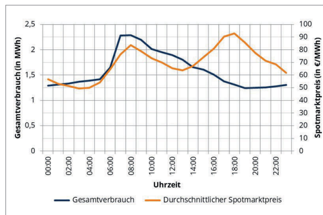
Bild 7. Verlauf des durchschnittlichen täglichen Gesamtverbrauchs und des Spotmarktpreises für den Winter 2024 der Baustelle E (Szenario 1). Grafik: IBB-TUD, Datengrundlage [16] Fig. 7. Course of average daily total consumption and spot market price for winter 2024 of construction site E (scenario 1). Source: IBB-TUD, data basis [16]
