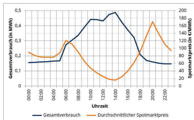
Bild 8. Verlauf des durchschnittlichen täglichen Gesamtverbrauchs und des Spotmarktpreises für den Sommer 2024 der Baustelle E (Szenario 1). Grafik: IBB-TUD, Datengrundlage [16] Fig. 8. Course of average daily total consumption and spot market price for summer 2024 of construction site E (scenario 1). Source: IBB-TUD, data basis [16]
