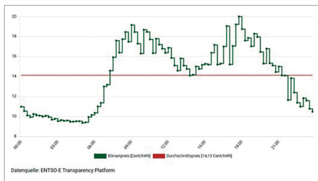
Bild 2. EPEX-Spot-Preise, exemplarisch für den 26.01.2026. Grafik: [16] Fig. 2. EPEX Spot prices, exemplary for 26.01.2026. Source: [16]
