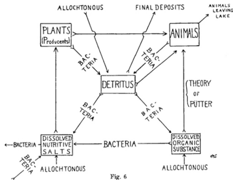
Abbildung 6.10 – Stoffwechselkreislauf in einem See
