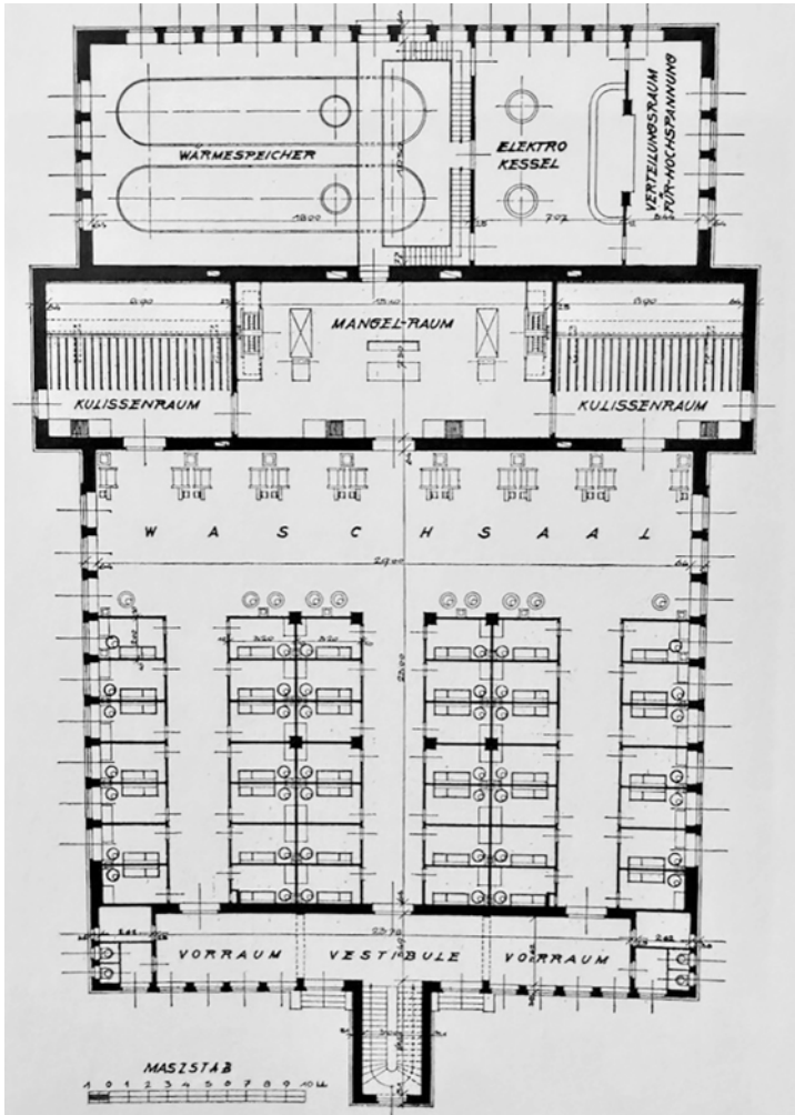
Abb. 20: Grundriss der großen Zentralwäscherei im Karl Marx-Hof.
