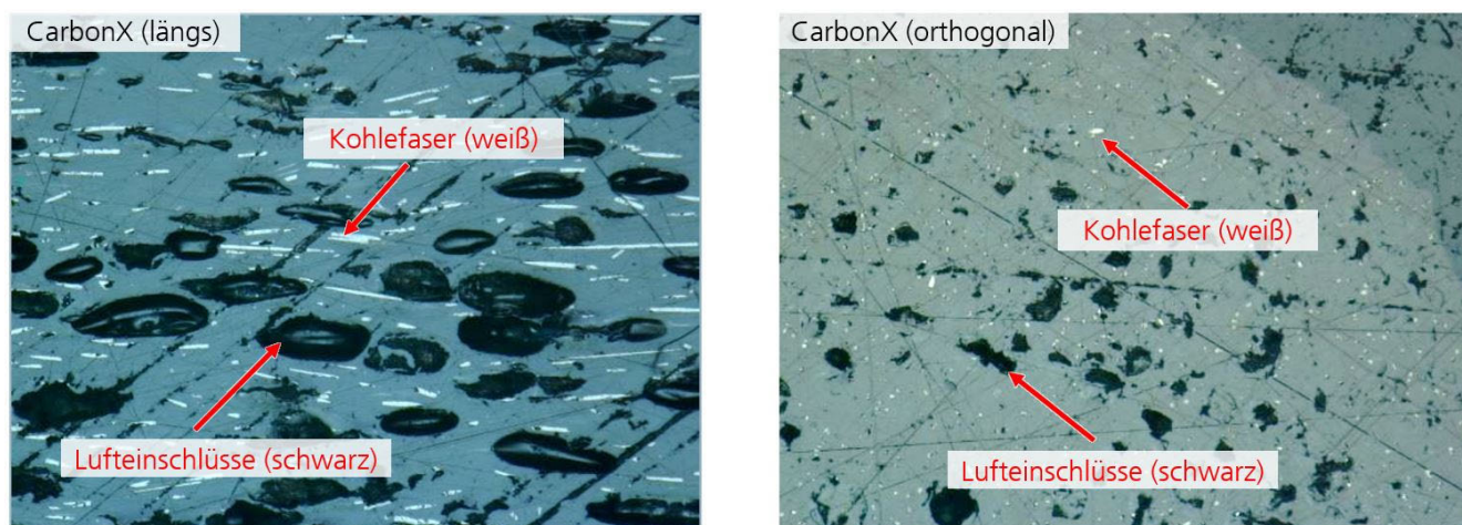
Bild 1. Schlichtbilder von „CarbonX ULTEM 1010“ Filament von 3DXtech (links: Längsschliff, rechts: Orthogonalschliff durch Filamentquerschnitt). Grafik: Fraunhofer IPA
