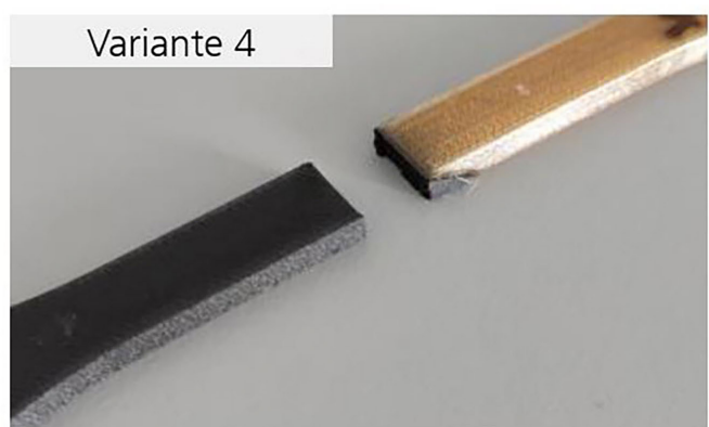
Bild 5. Charakteristisches Bruchbild der unterschiedlichen Verbindungsvarianten (schwarz: fasergefülltes Material, goldbraun: ungefülltes Material). Grafik: Fraunhofer IPA
