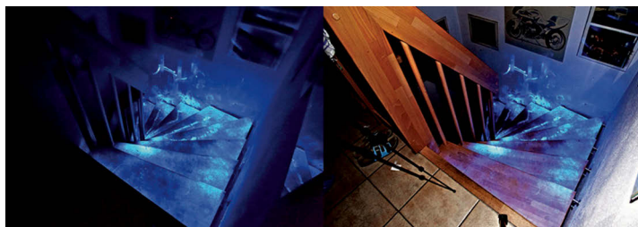
Abb. II.6: Integration von 2D-Luminolaufnahmen in den Laserscan:
