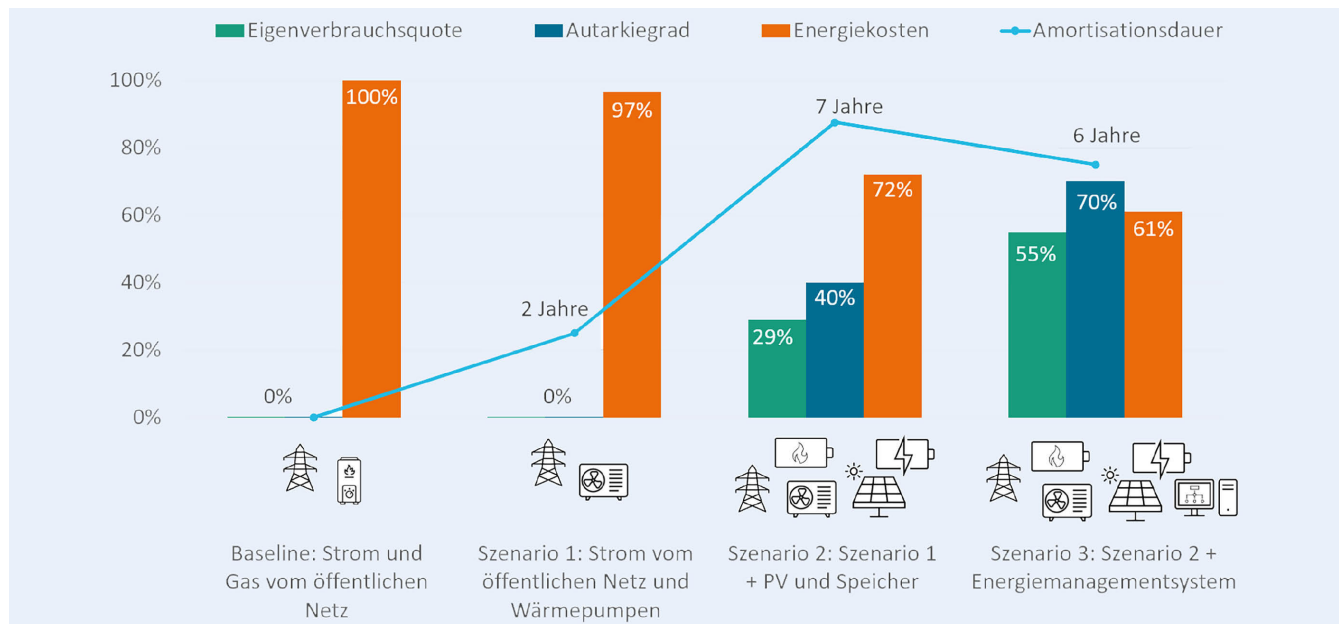
Bild 3. Ergebnisse des Szenarienvergleichs. Grafik: Fraunhofer IPA
