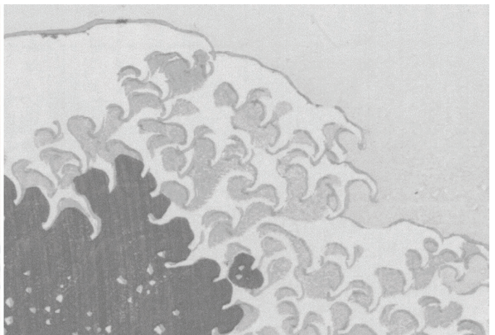
9 »Die Große Welle«, Bayerische Staatsbibliothek, Res/4 L.jap. K 408, Detail: Vergleich der Vis (sichtbares Licht)- mit der Infrarot (940 nm)-Aufnahme: Indigo wird transparent, Preußisch Blau bleibt sichtbar Abb.: Bayerische Staatsbibliothek / IBR
