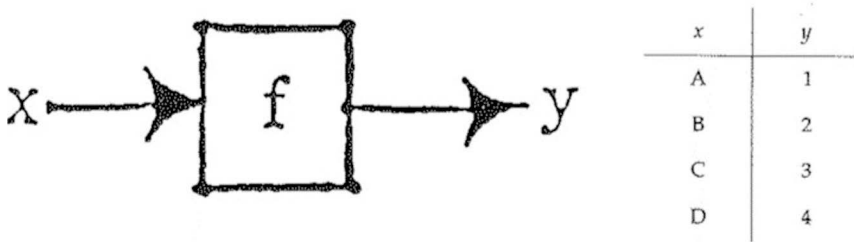
Abb. 1: Triviale Maschine 65
