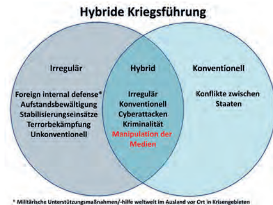
Abb.IV.2 Konzeptionelles Modell Hybrider Kriegführung
