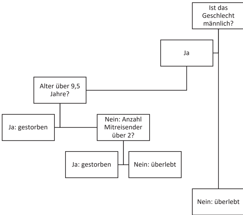
Abb. 10: Einfacher Entscheidungsbaum 375
