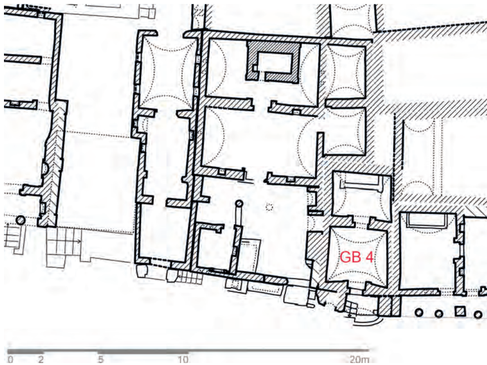
Abb. 2: Grundriss Erdgeschoss; 2021
