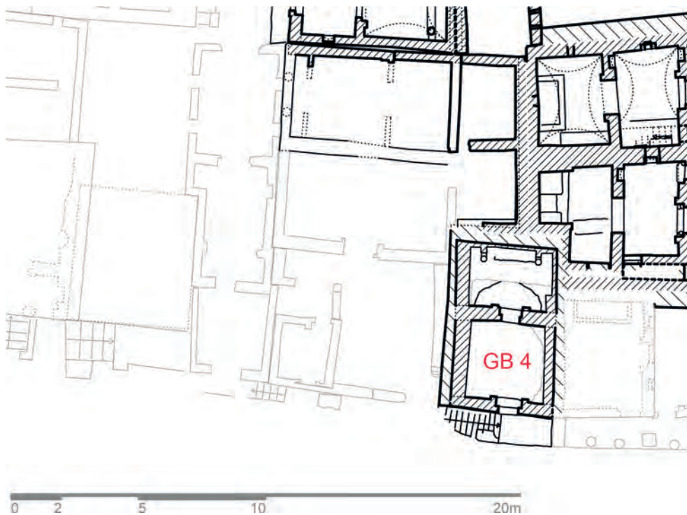
Abb. 3: Grundriss Obergeschoss; 2021
