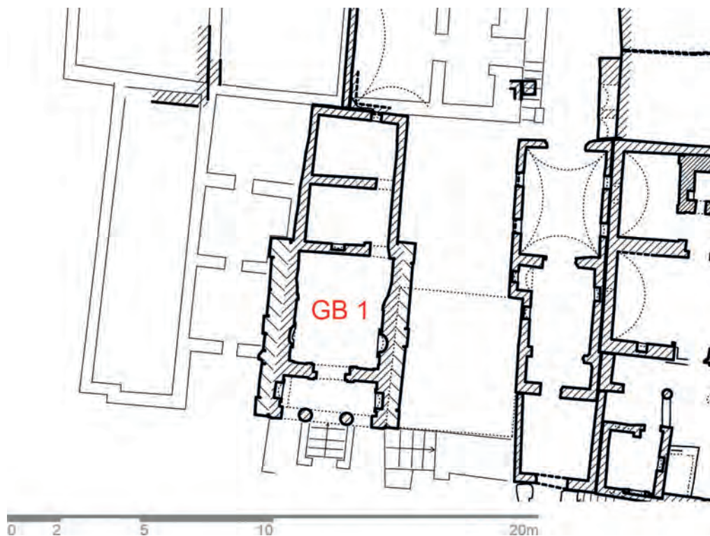
Abb. 2: Grundriss; 2021
