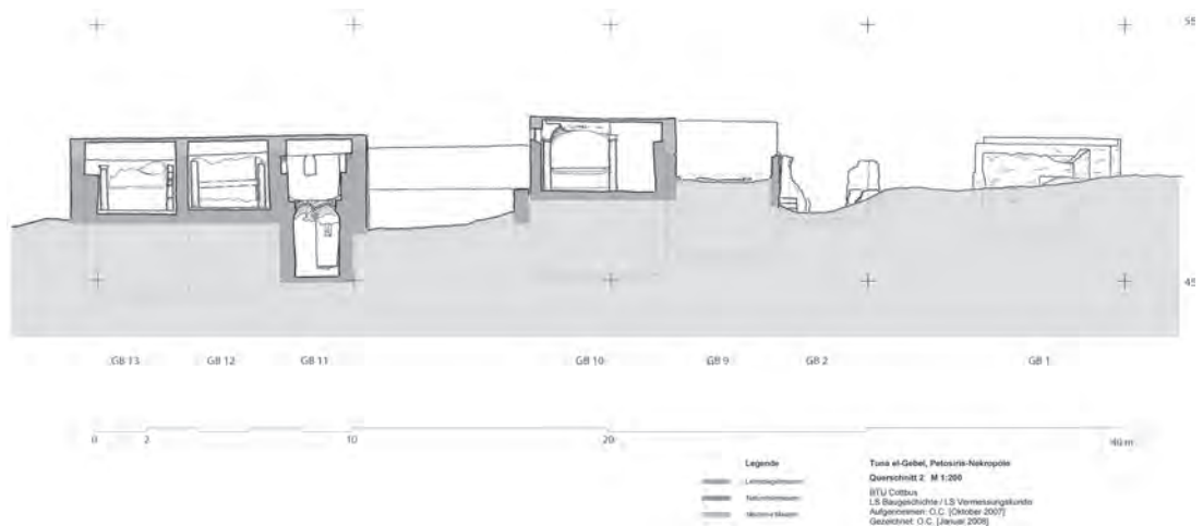
Abb. 11: Querschnitt von GB 13 (im Osten) bis GB 1 (im Westen); 2008
