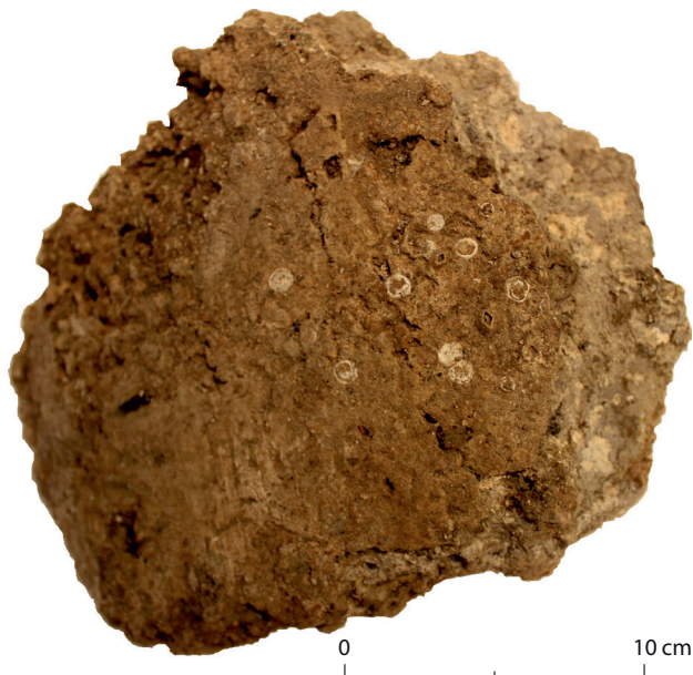
Abb. 12. Wrack am Stülper Huk. Entnommenes Fragment der Ladung, welches analysiert wurde. Auf der Oberfläche sind die Spuren der vergangenen Holzdauben sowie Seepocken ( semibalanus balanoides ) sichtbar (Foto: F. Jürgens/CAU Kiel).
