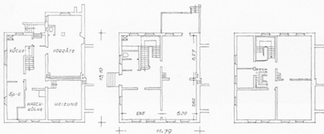
Abb. 148. Keller-, Erd- und Obergeschoßgrundriß des Kopfbaues der gleichen Hausreihe
