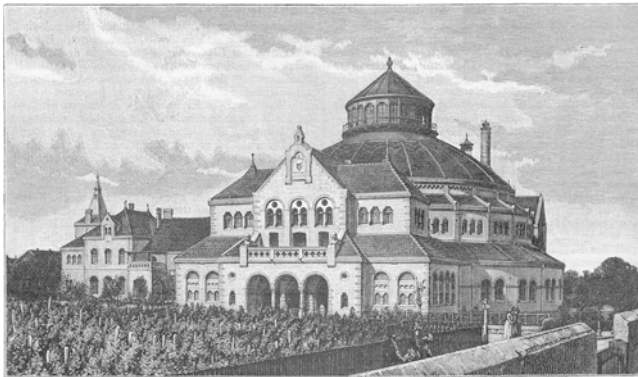
Abb. 67 Otto March, Volksbühne Worms, Städtisches Volkstheater und Festhaus, Worms, 1888–1889. Ansicht (oben) und Grundriss (unten)
