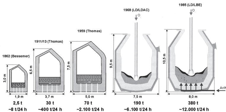
Abb. 6: Entwicklung der Konvertergrößen und Durchsatzleistungen 1892–1985 106
